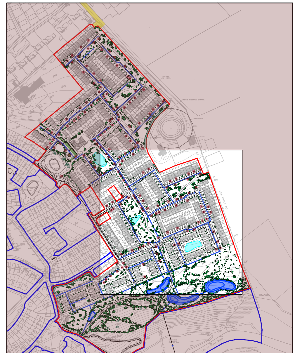
Site Layout - Key Plan Scale: 1:5000
